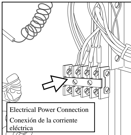
Figure 6 Main Terminal Block Bloque terminal eléctrico
