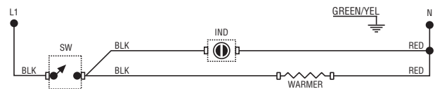
SCHEMATIC WIRING DIAGRAM WX1A
