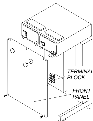
Fig. 3 115/230 Volt Terminal Block
