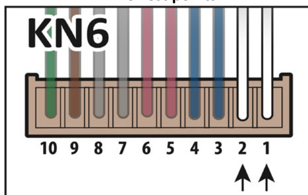
E3 Test points
