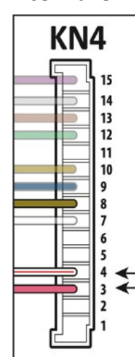
E9 Test points Ice Maker 2
