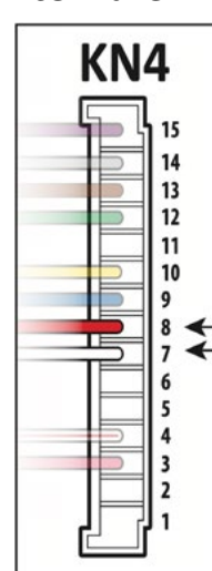
E9 Test points Ice Maker 1
