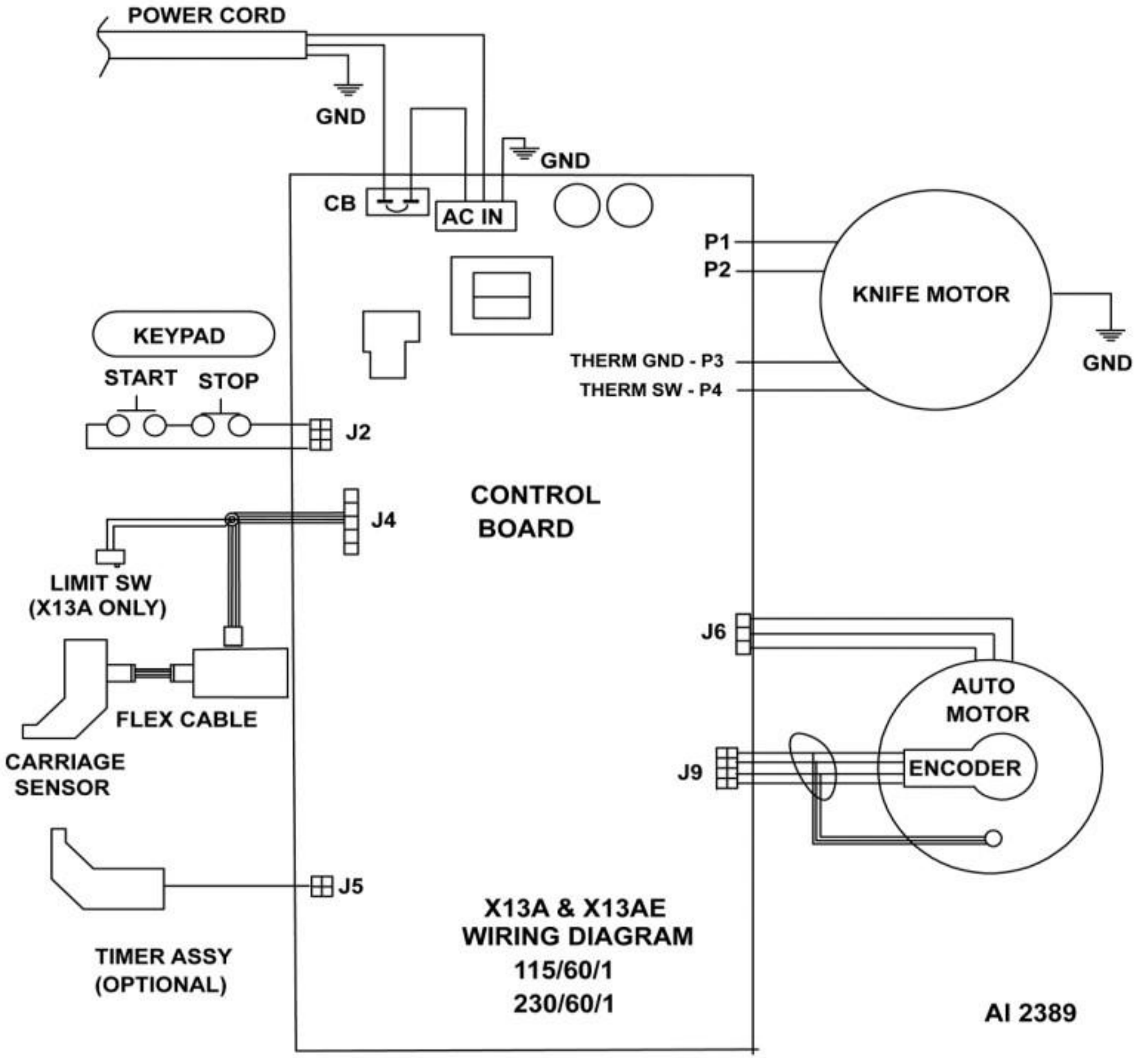
X13A & X13AE Wiring Diagram
