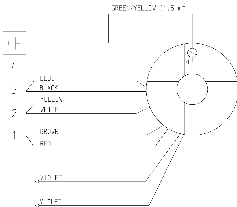
FAN MOTOR CONNECTIONS
