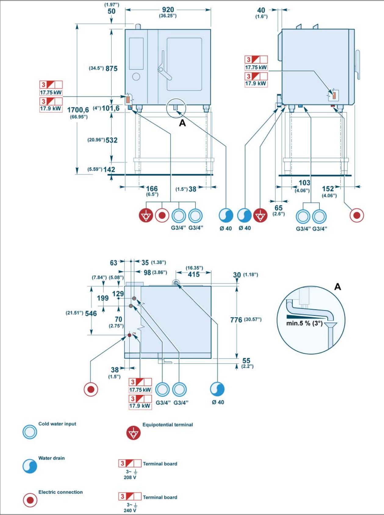
OVEN CONNECTION DIAGRAM (FX 101 E3 - FX 101 E3C)
