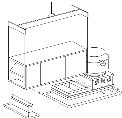
Installation de l'unité d'alimentation
