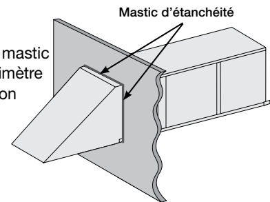
Scellement de l'ouverture murale
